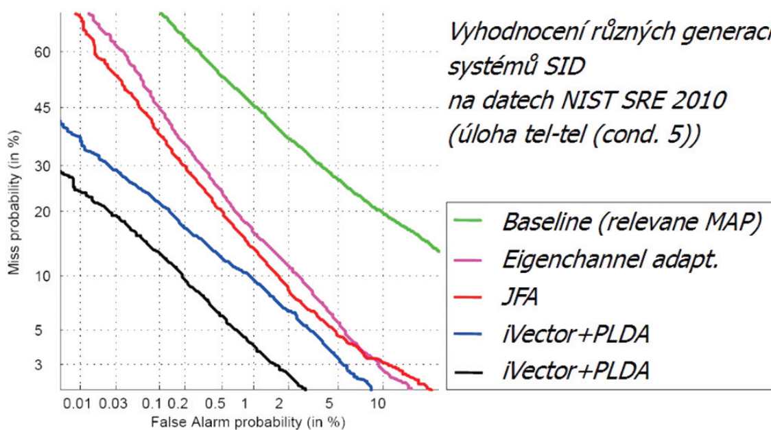
Obrázek 3 – Příklad znázornění přesnosti systémů rozpoznání řečníka s využitím různých algoritmů
