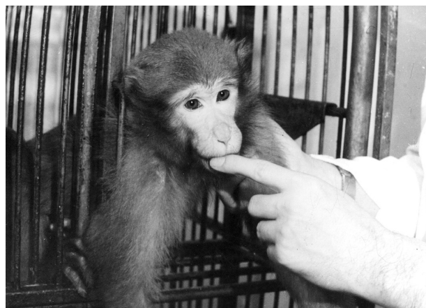
Obr 3 – Imobilizace makaka rhesus ( Macaca mulatta ) carfentanilem v dávce 2 \mu\text{g}/\text{kg} i.m. Úplná ztráta agresivního chování (Zdroj: archiv autora)
